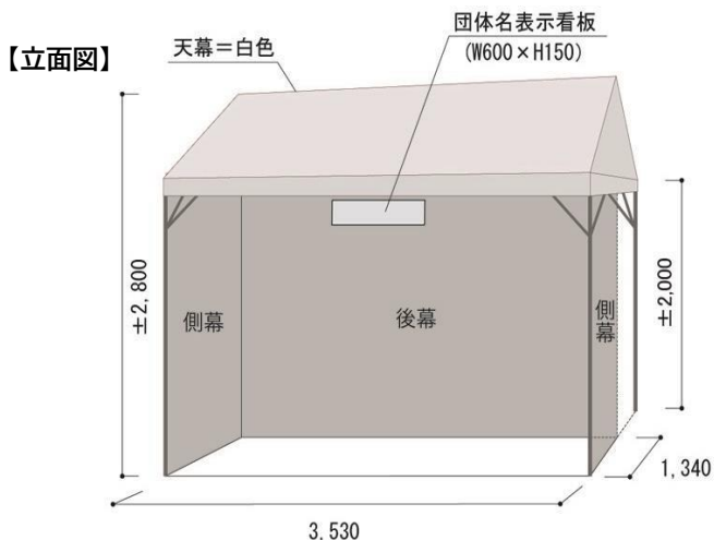
【立面図】
